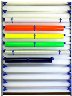
Rollenregal (ca. 200 cm hoch) – Wandmontage (6 Befestigungspunkte) vorbereitet für 12 Rollen
